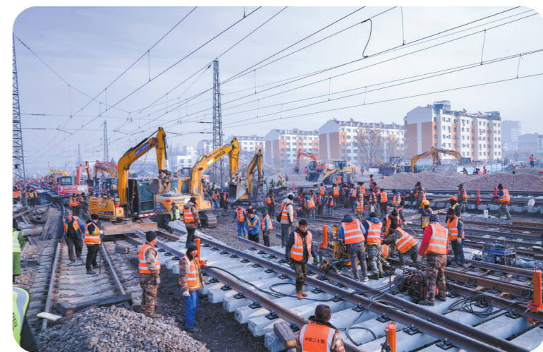
图为包(头)银(川)高铁乌海站站场改造施工现场
